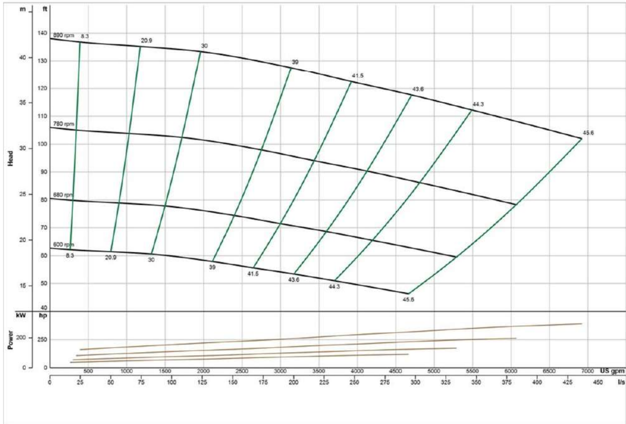
EDDY Pump – EXF12K Accesorio Hidráulico para Excavadora – Curva de la
