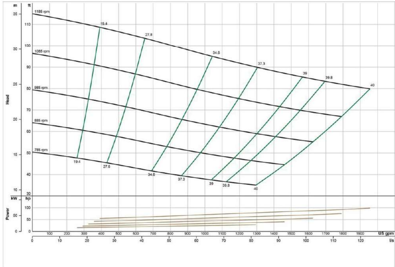
EDDY Pump – EXF6K Accesorio Hidráulico para Excavadora – Curva de la Bomba
